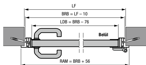
Mellékajtó alumínium saroktokkal, 2. profiltípus Belülre szerelt
