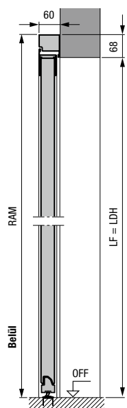
Mellékajtó alumínium blokkokkal, 2. profiltípus Beépítés a nyílás mögé
