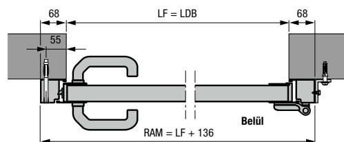
Mellékajtó alumínium blokkokkal, 2. profiltípus Beépítés a nyílás mögé
