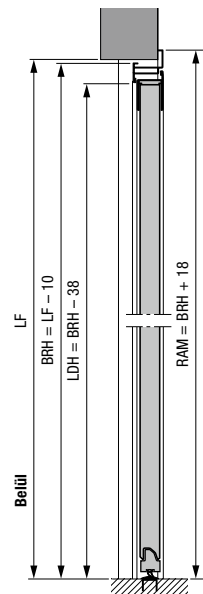
Mellékajtó alumínium saroktokkal, 2. profiltípus Kívülre szerelt
